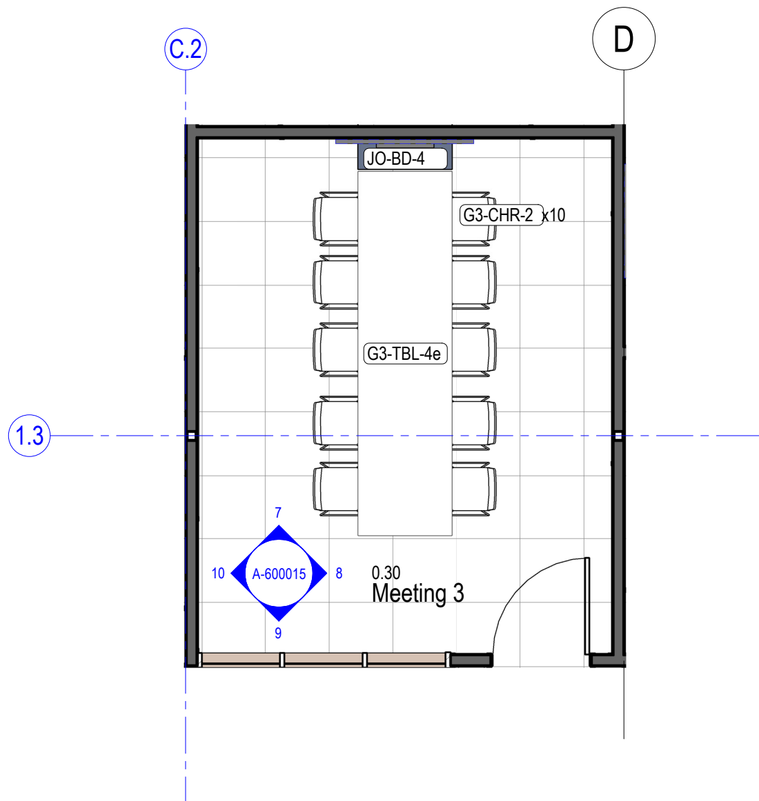
6 0.30 - Meeting 3 - Plan 1 : 50
